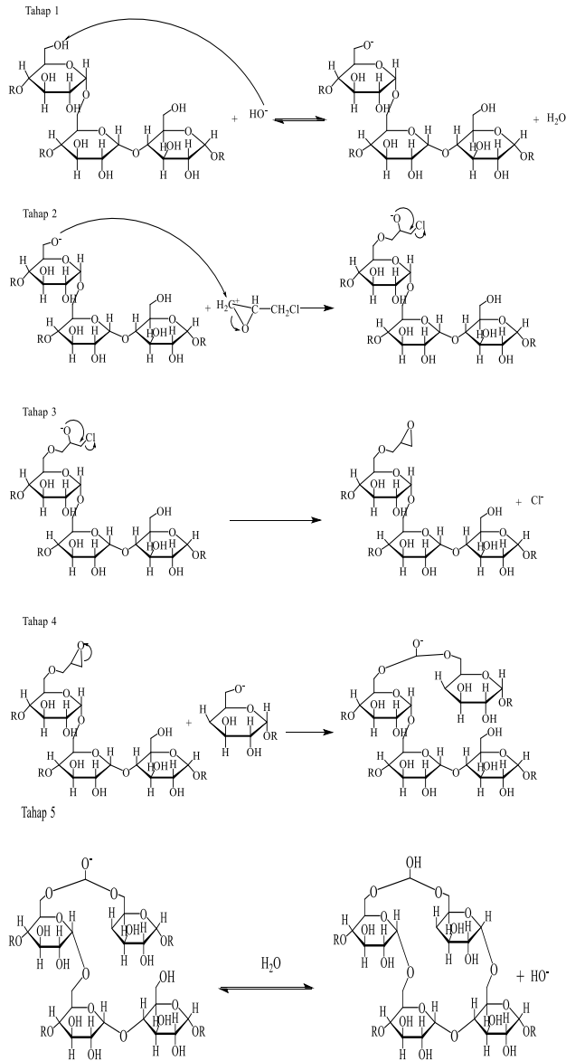
Gambar 3. Reaksi sintesis pati-epiklorohidrin (Kim et al., 2002).
